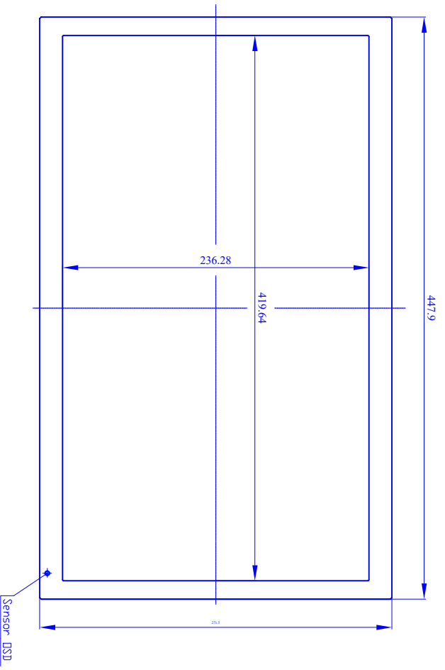
FRONTANSICHT
